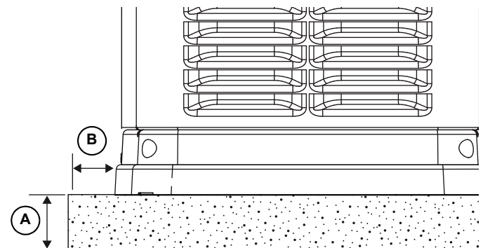
Figure 3-3. Terre compactée ou gravier
