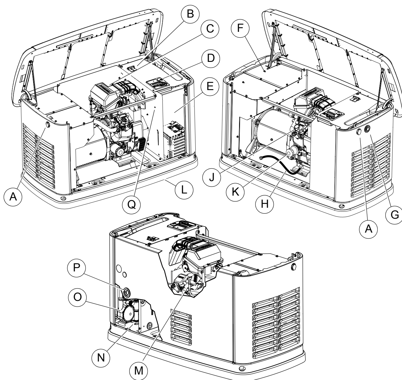
Figura 2-2. 11 kW–22 kW—Ubicaciones de componentes y control
