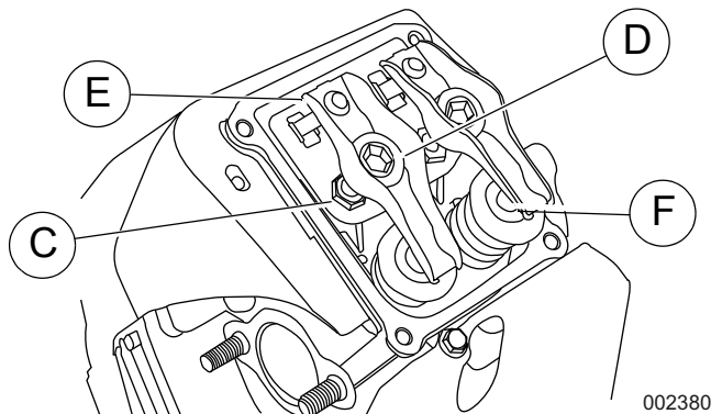
Figura 4-8. Ajuste de la luz de válvulas (11-22 kW)
