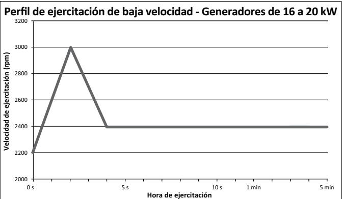
Figura 3-9. Perfil de ejercitación de baja velocidad (16-20 kW)
