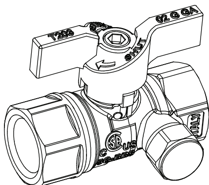
Figura 5-2. Válvula de accesorio con lumbrera para manómetro
