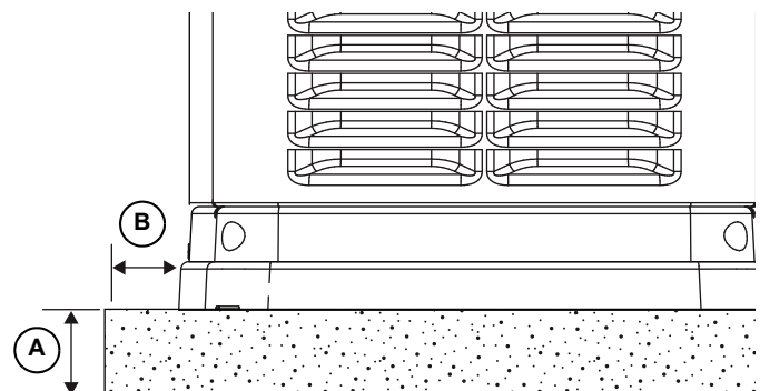
Figura 3-3. Basamento de gravilla o suelo compactado
