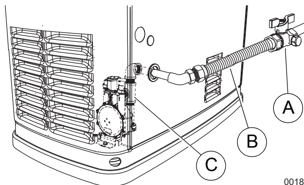
Figura 5-3. Colector de sedimentos, válvula de cierre de combustible con lumbrera del manómetro y tubería de combustible flexible
