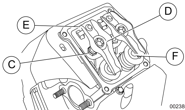
Figura 4-4. Ajuste de la luz de la válvula
