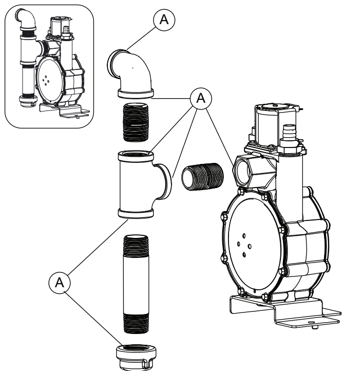
Figure 4-7. Vérification des fuites aux points de raccordement
