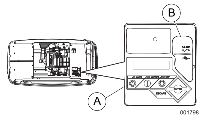
Figure 3-6. Panneau de commande du générateur
