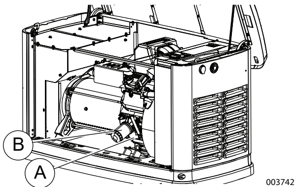
Figure 4-1. Emplacement du filtre à huile et du point de vidange
