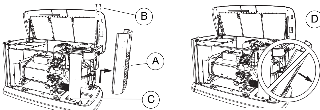
Figure 3-4. Retrait du panneau latéral d'admission
