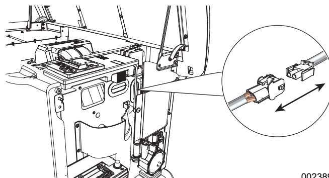
Figure 4-8. Débranchez le câble du chargeur de la batterie
