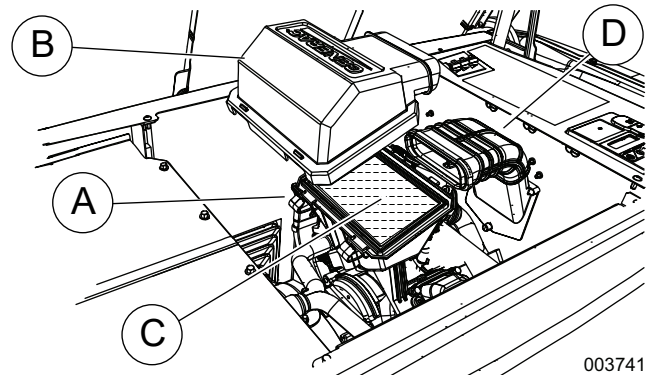
Figure 4-2. Entretien du filtre à air
