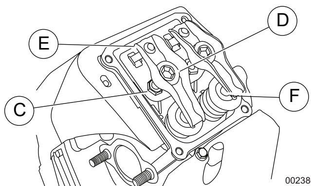
Figure 4-4. Réglage du jeu de soupapes
