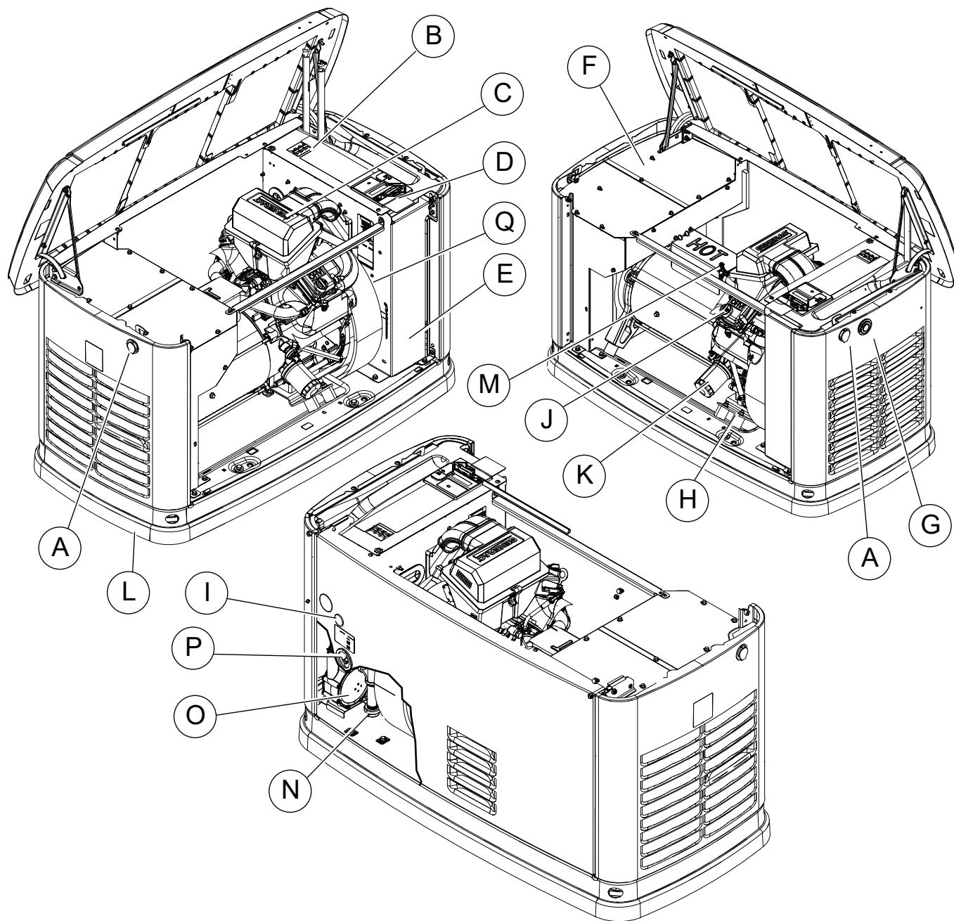
Figure 2-1. Emplacements des composants et des commandes
