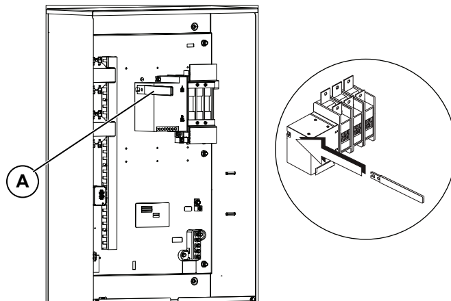
Figure 3-10. Actionnement manuel type du commutateur de transfert
