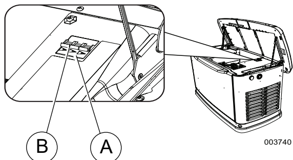
Figure 3-2. Disjoncteur principal
