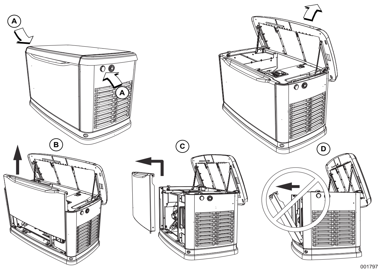
Figure 3-3. Emplacement des loquets latéraux et procédure de retrait du panneau avant
