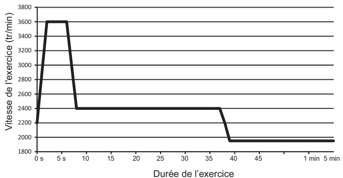
Figure 3-9. Profil du moteur à basse vitesse durant un cycle d'exercice
