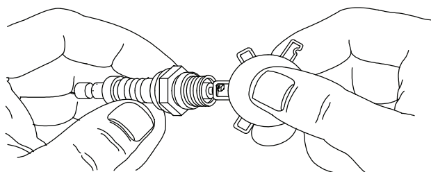
Figure 4-3. Mesure de l'écartement des bougies d'allumage
