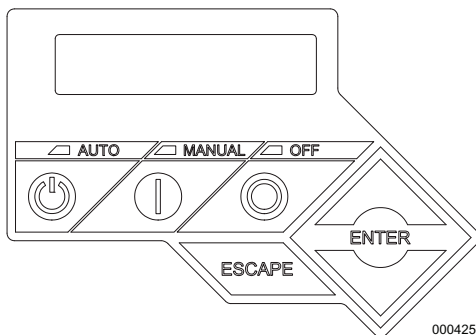
Figura 7-1. Panel de control del generador
