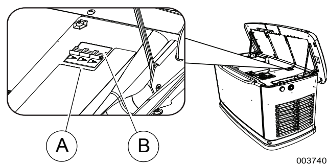
Figura 2-8. Disyuntor de la línea de alimentación del generador
