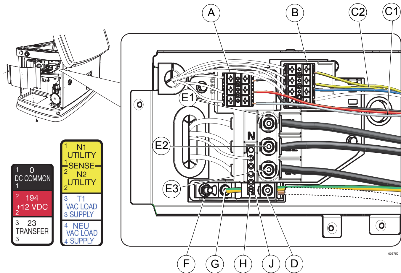
Figura 6-1. Conexiones de cableado eléctrico
