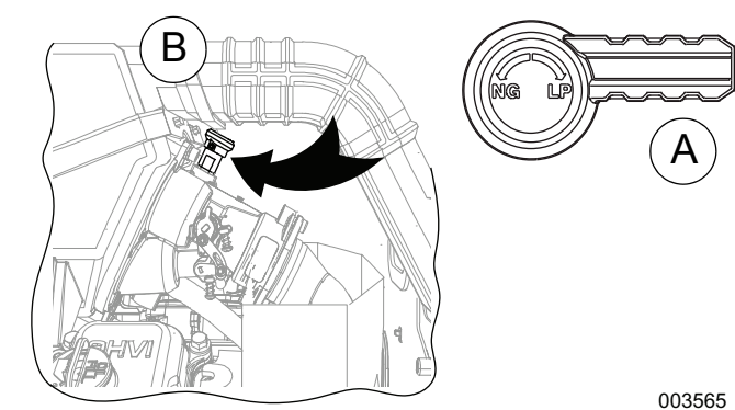
Figura 5-1. Ubicación del mando de conversión del combustible
