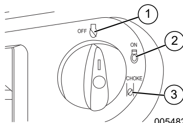
Figure 2-5. Commutateur (exemple)
