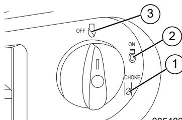
Figure 3-2. Positions OFF/ON/CHOKE (Arrêt/Marche/Étranglement)
