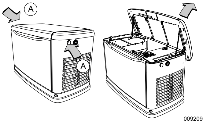
Figure 2-4. Ouvrir le capot supérieur
