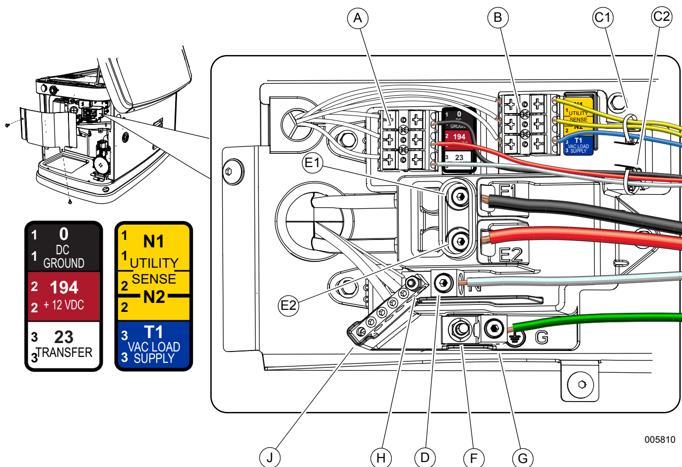
Figure 6-1. Raccordements électriques
