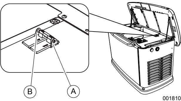
Figure 2-9. Disjoncteur principal de la génératrice (MLCB)
