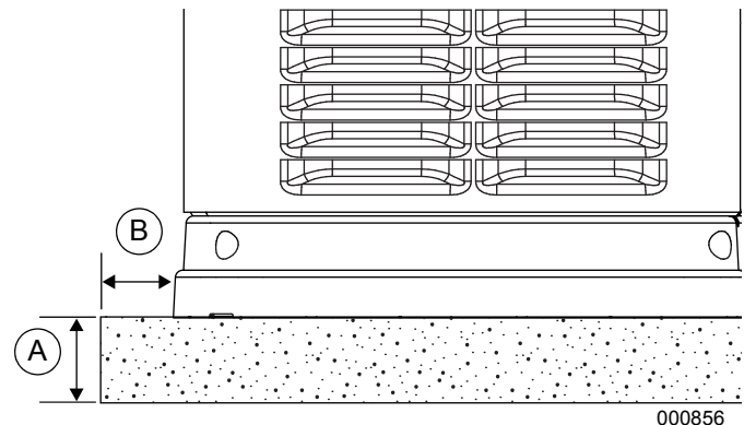
Figure 3-4. Surface d'appui en gravier ou dalle en béton
