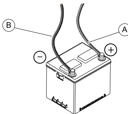
Figure 6-2. Raccordement des câbles de batterie
