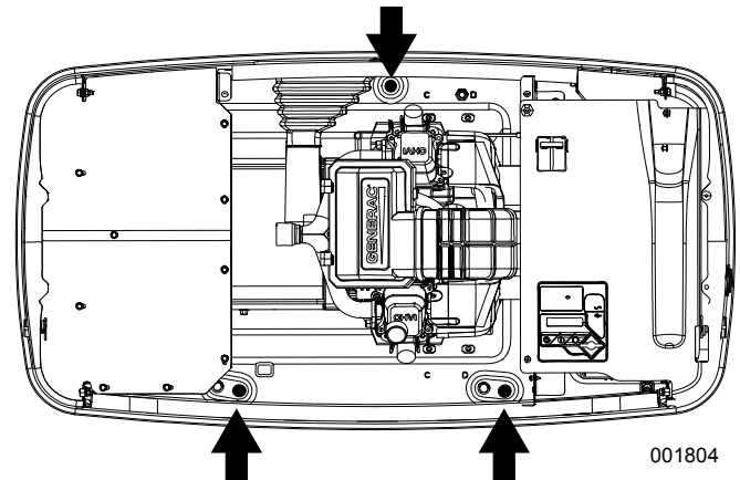
Figure 4-2. Emplacement des trous de fixation
