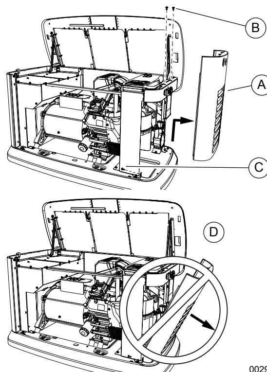
Figure 2-6. Dépose du panneau latéral d'admission
