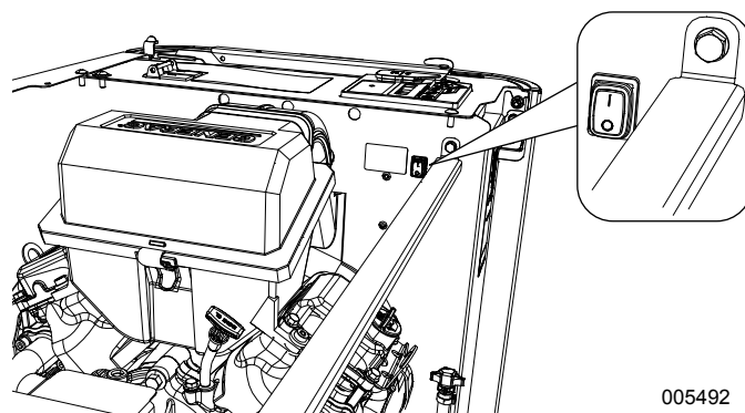
Figure 2-12. Interrupteur d'arrêt auxiliaire (13-22 kW)
