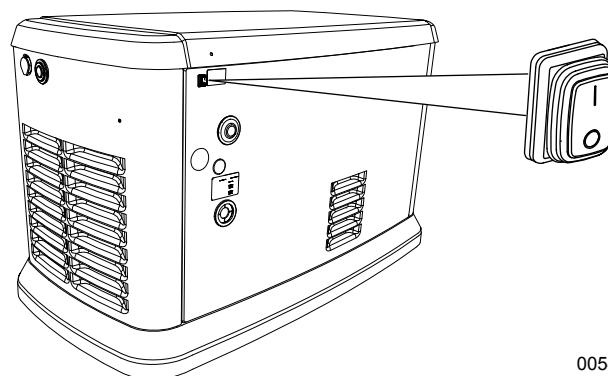
Figure 2-11. Interrupteur d'arrêt auxiliaire (tous les modèles)
