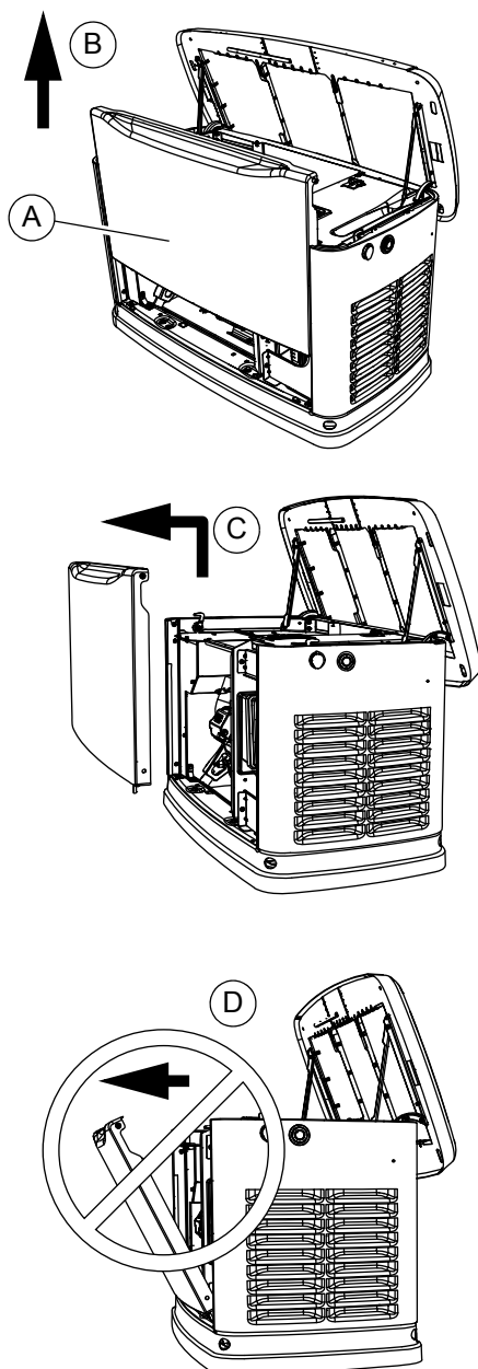
Figure 2-5. Déposer le panneau d'accès avant
