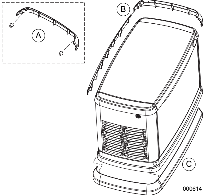
Figure 4-3. Pose de la bordure de socle
