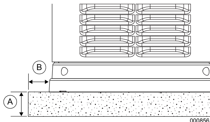
Figura 3-4. Grava compactada o losa de hormigón
