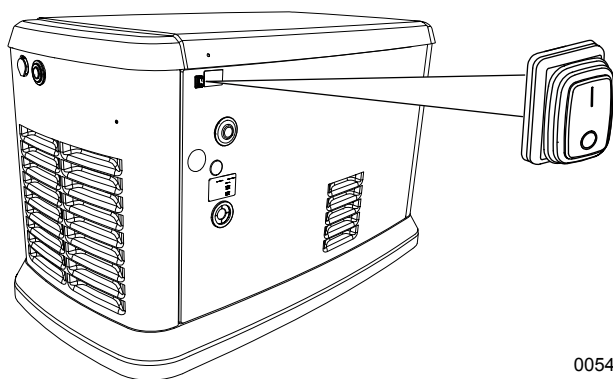
Figura 2-11. Interruptor de desconexión auxiliar (todos los modelos)
