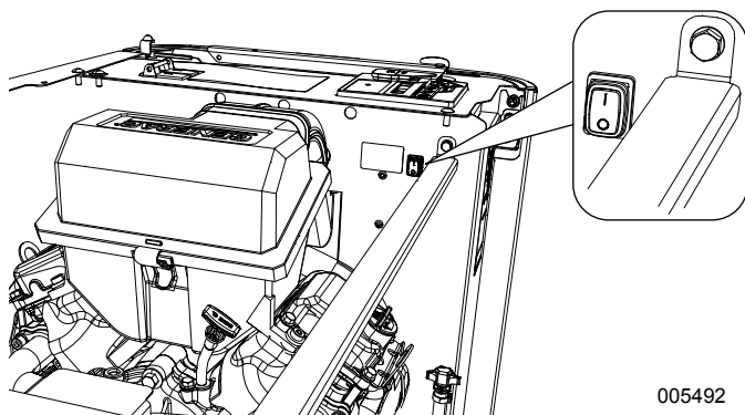
Figura 2-12. Interruptor de desconexión auxiliar (13 a 22 kW)
