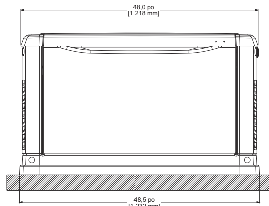
VUE AVANT
