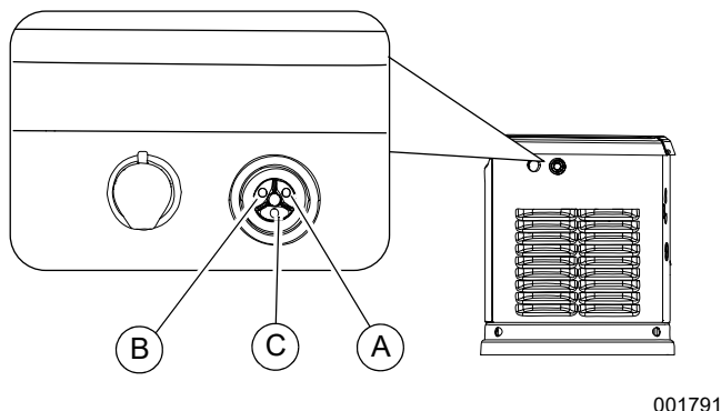
Figure 3-5. Voyants indicateurs
