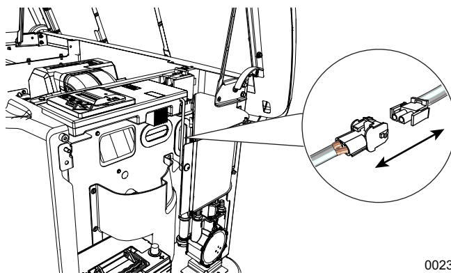
Figure 4-9. Débrancher le câble de chargeur de batterie
