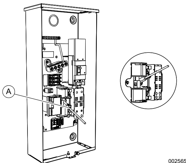
Figure 3-11. Fonctionnement d'un commutateur de transfert manuel typique
