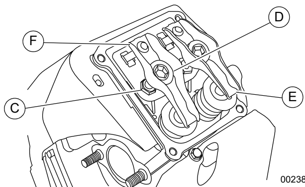
Figure 4-8. Réglage du jeu des soupapes (20 à 24 kW)
