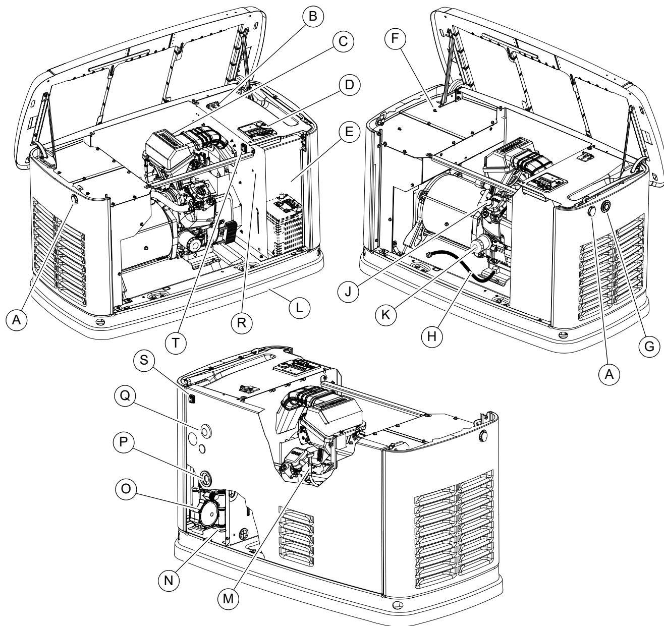
Figure 2-3. 20 kW à 24 kW — Emplacement des composants et des commandes
