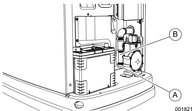
Figure 4-11. Nettoyer le piège à sédiments
