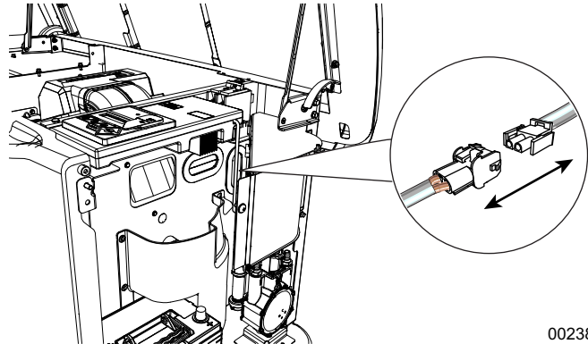
Figura 4-9. Desconexión del cable del cargador de la batería
