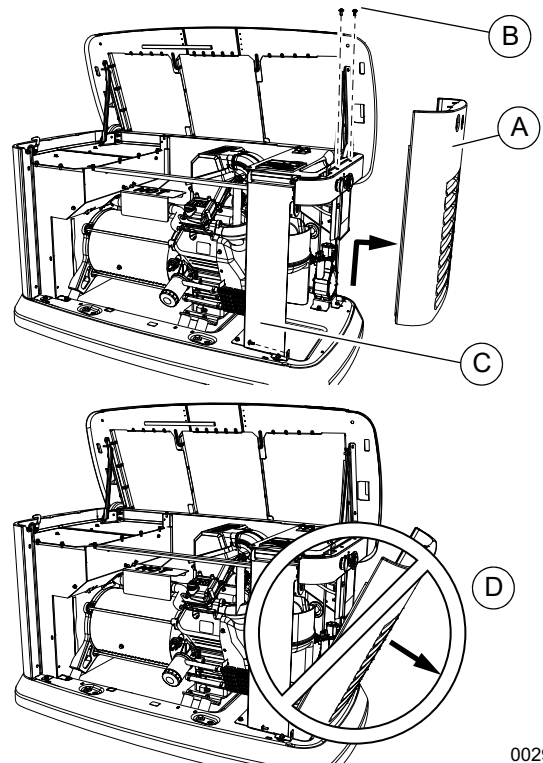
Figura 3-3. Retiro del panel lateral de entrada
