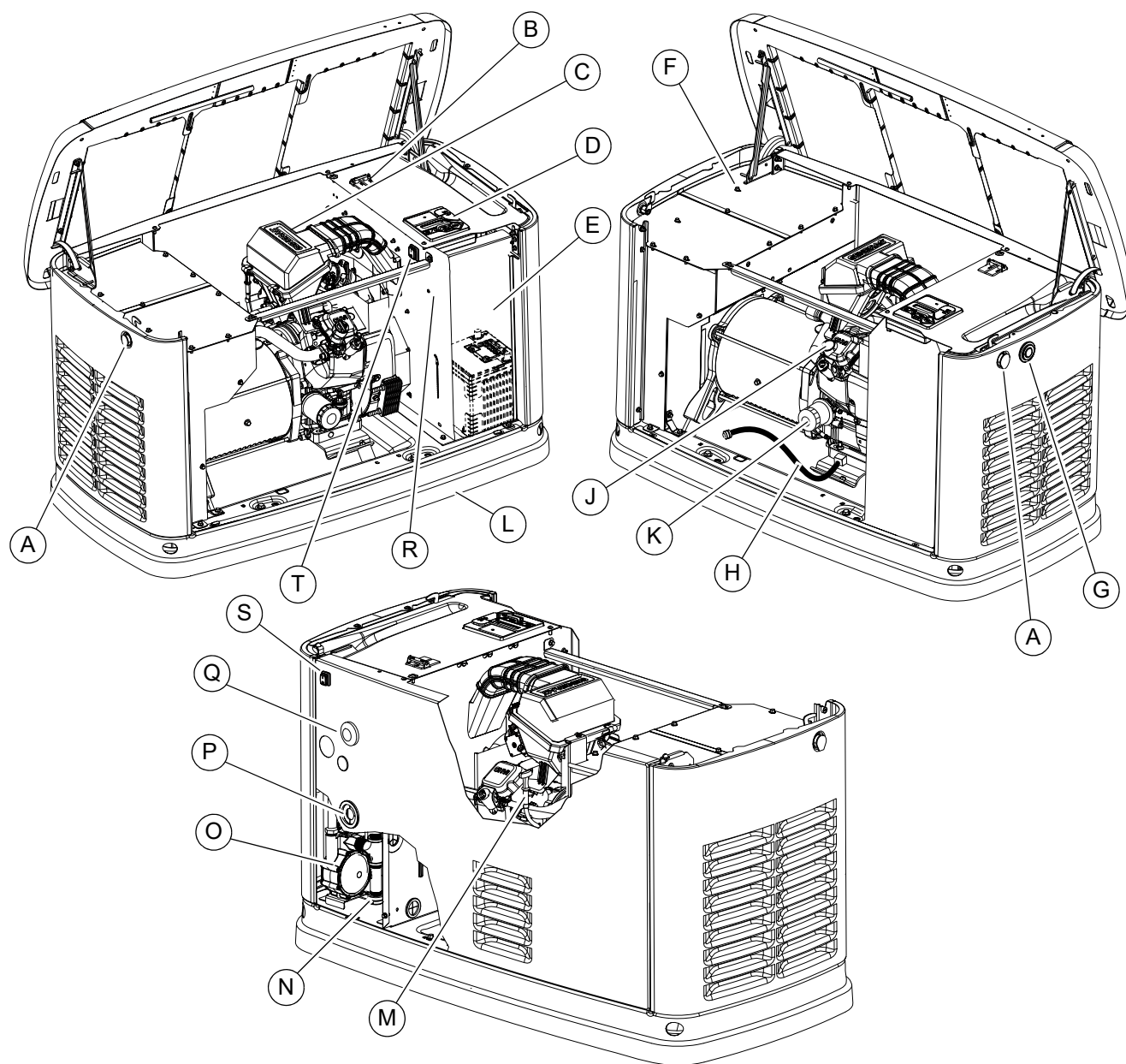
Figura 2-3. 20 kW a 24 kW—Ubicaciones de controles y componentes
