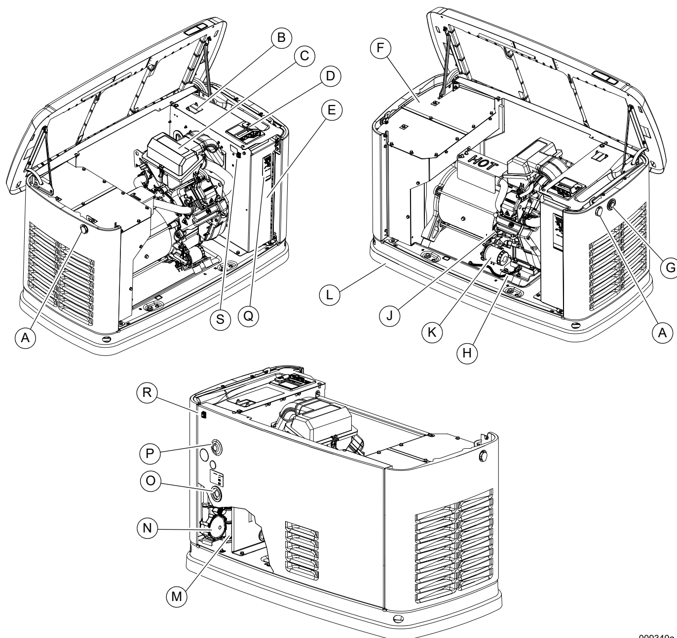
Figura 2-2. 14 kW a 18 kW—Ubicaciones de controles y componentes
