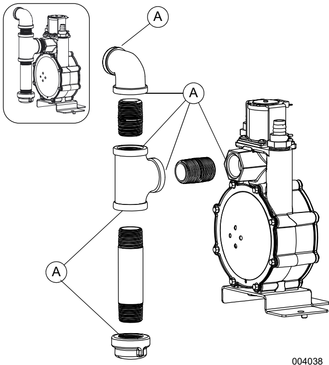
Figura 4-12. Comprobación de fugas en los puntos de conexión
