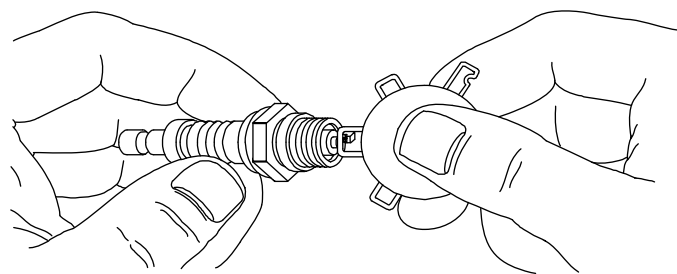
Figura 4-6. Medición de la separación de las bujías
