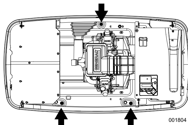
Figure 4-2. Emplacement des trous de fixation
