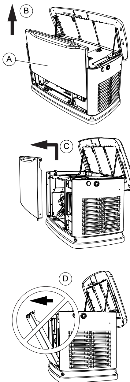
Figure 2-5. Déposer le panneau d'accès avant
