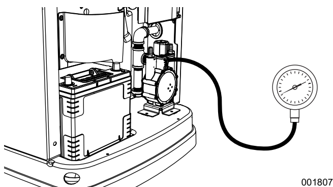
Figure 5-4. Contrôle de pression au manomètre
