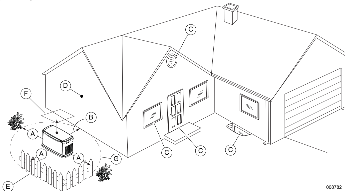
Figure 3-2. Distances requises de séparation du générateur
