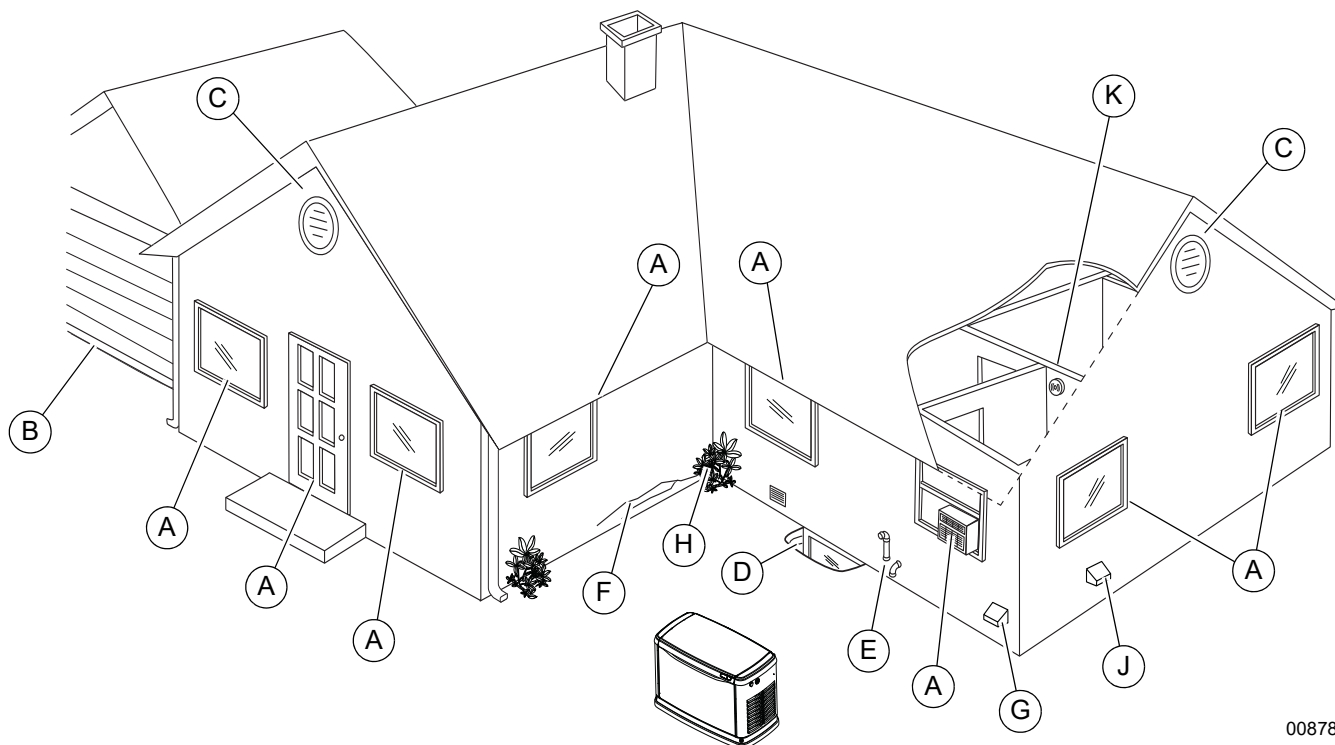
Figure 3-1. Monoxyde de carbone — Points d'entrée potentiels
