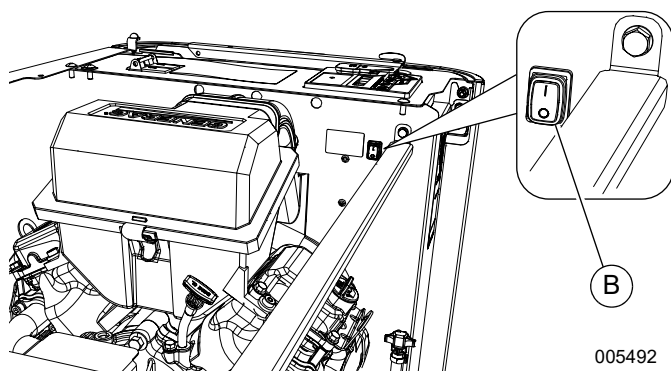
Figure 2-12. Interrupteur d'arrêt auxiliaire (14-24 kW)
