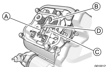
Figure 4-7. Réglage du jeu des soupapes (10 kW)
