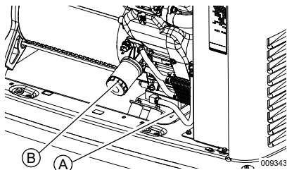
Figure 4-3. Emplacement de filtre à huile et flexible de vidange (20 à 26 kW)
