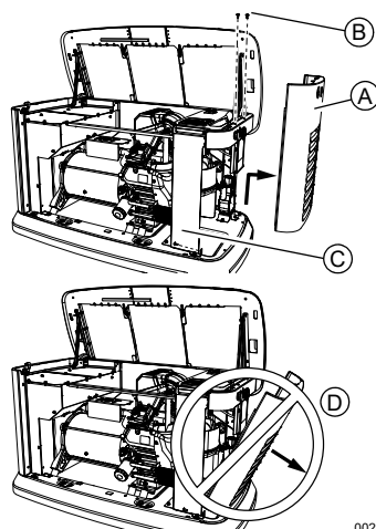
Figure 3-3. Dépose du panneau latéral d'admission
