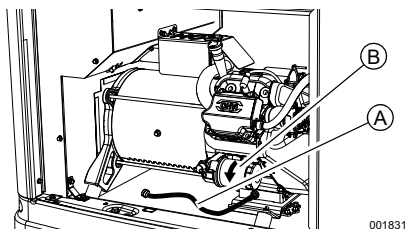
Figure 4-1. Emplacement de filtre à huile et flexible de vidange (10 kW)
