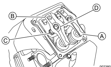
Figure 4-8. Réglage du jeu des soupapes (20 à 26 kW)
