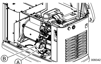
Figure 4-2. Emplacement de filtre à huile et flexible de vidange (14 à 18 kW)
