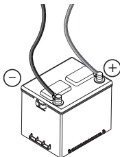
Figura 4-10. Cables de la batería
