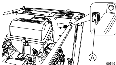
Figura 3-7. Interruptor de desconexión de emergencia interno (14 a 26 kW)
