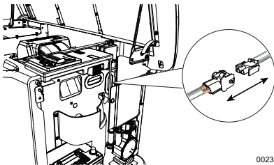
Figura 4-9. Desconexión del cable del cargador de la batería
