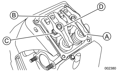
Figura 4-8. Ajuste de la separación de la válvula (20 a 26 kW)
