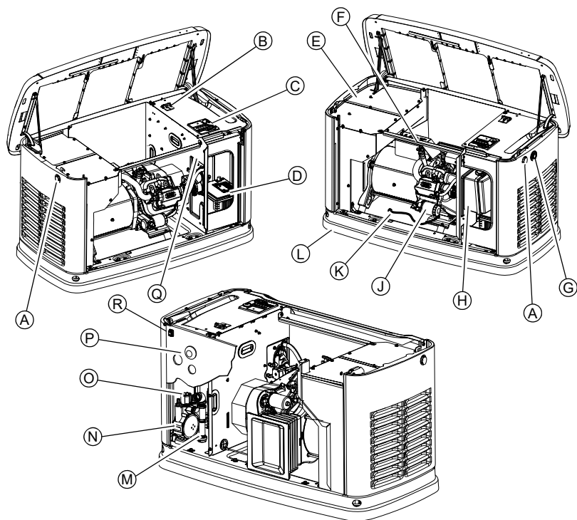
Figura 2-1. 10 kW—Ubicaciones de controles y componentes
