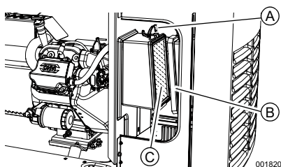
Figura 4-4. Mantenimiento del filtro de aire (10 kW)
