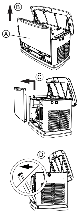
Figura 3-2. Retiro del panel de acceso delantero
