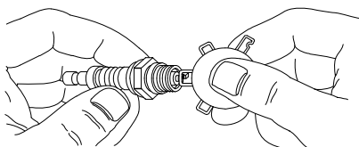
Figura 4-6. Medición de la separación de las bujías
