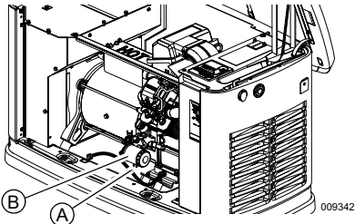
Figura 4-2. Ubicación del drenaje y filtro de aceite (14 a 18 kW)
