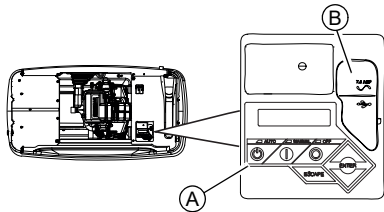
Figura 3-8. Panel de Control del generador
