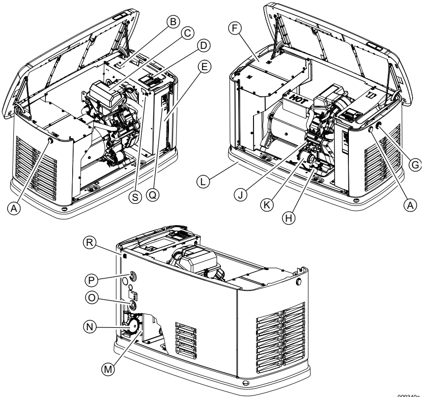
Figura 2-2. 14 kW a 18 kW—Ubicaciones de controles y componentes
