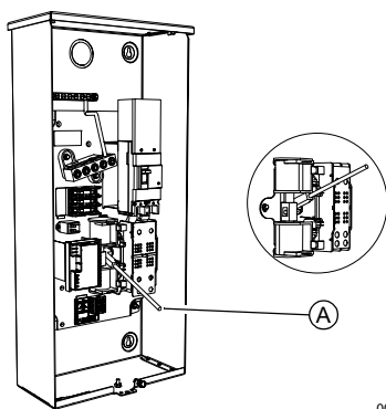
Figura 3-11. Funcionamiento del interruptor de transferencia manual típico
