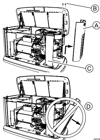
Figura 3-3. Retiro del panel lateral de entrada
