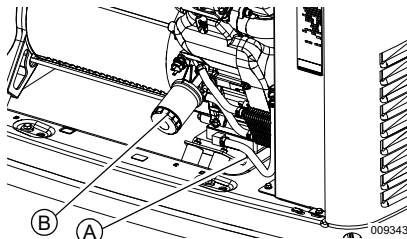
Figura 4-3. Ubicación del drenaje y filtro de aceite (20 a 26 kW)
