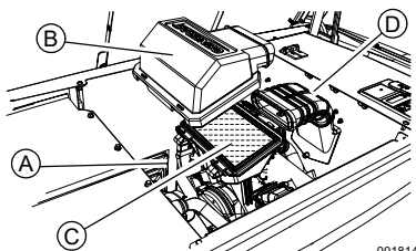
Figura 4-5. Mantenimiento del filtro de aire (14 a 26 kW)
