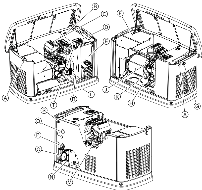
Figura 2-3. 20 kW a 26 kW—Ubicaciones de controles y componentes
