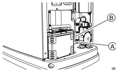
Figura 4-11. Limpieza del colector de sedimentos
