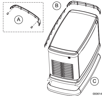
Figura 4-3. Instalación de la carcasa
