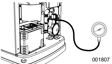
Figura 5-4. Revisión de la presión con manómetro
