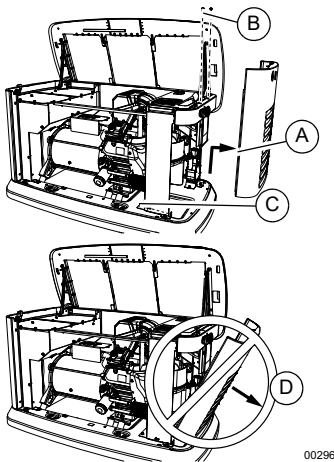
Figura 2-5. Retiro del panel lateral de entrada
