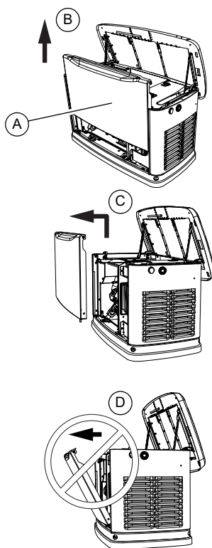
Figura 2-4. Retiro del panel de acceso delantero
