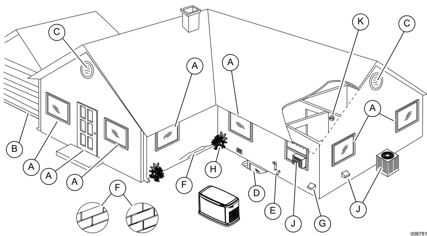
Figura 3-1. Monóxido de carbono—Posibles puntos de entrada
