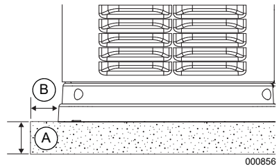
Figura 3-4. Gravilla o piedra triturada
