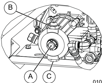
Figura 4-6. Vaciado/Llenado del aceite
