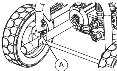
Figura 3-9. Aflojar el soporte de la cubeta
