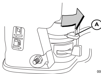
Figura 3-6. Válvula de combustible y cebador
