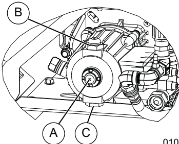
Figure 4-6. Vidange/Remplissage de l'huile
