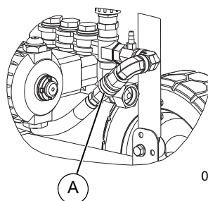
Figure 4-15. Déconnexion du tuyau de pompe
