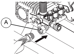
Figure 2-7. Inspection de la crépine d'admission et raccordement du tuyau d'alimentation en eau
