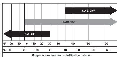
Figure 4-9. Viscosité de l'huile
