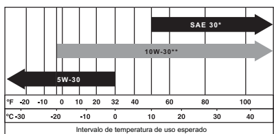
Figura 4-9. Viscosidad del aceite
