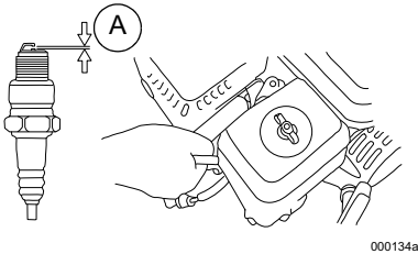
Figure 4-13. Bougie d'allumage
