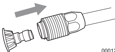
Figura 2-12. Insertar boquilla
