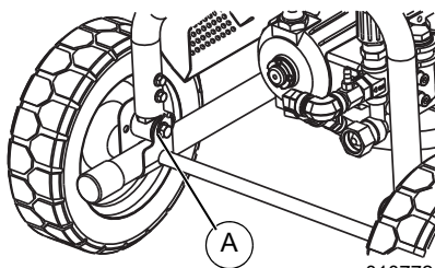
Figure 3-9. Déblocage du porte-seau
