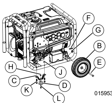
Figura 2-8. Ensamblaje de la rueda y la pata
