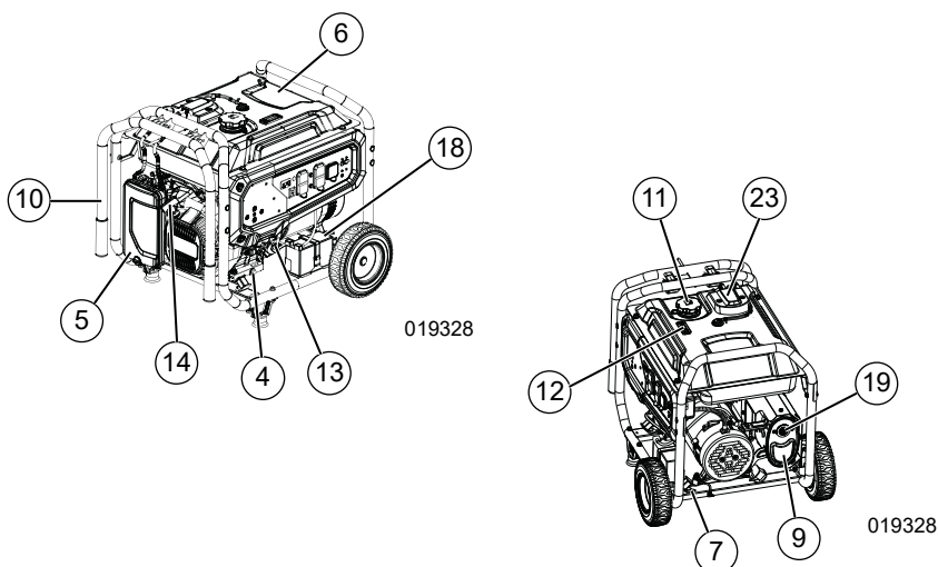
Figura 2-1. Características y controles
