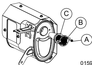
Figura 4-6. Pantalla del supresor de chispas
