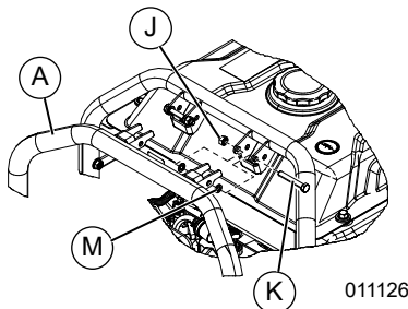
Figura 2-9. Ensamblaje de la manija
