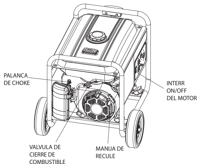
Figura 11 - Controles del motor
