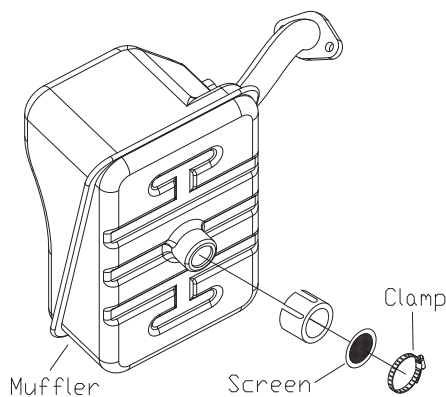
Figura 14 - Supresor de chispa
