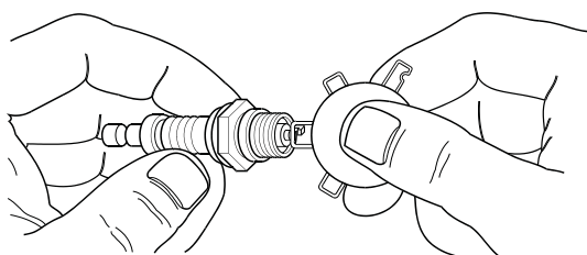
Figura 13 - Espaciado de la bujía.
