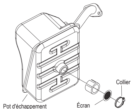
Schéma 14 - Pare-étincelles
