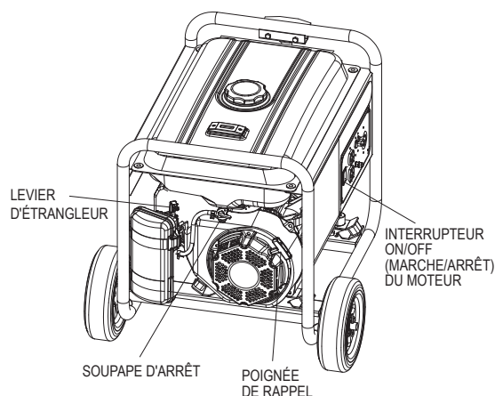
Schéma 11 - Commandes du moteur
