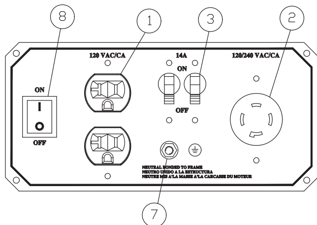
Schéma 3 - Panneau de commande
