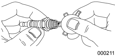
Figure 4-4. Bougie d'allumage
