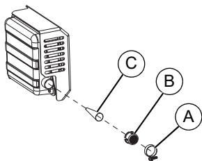
Figura 4-5. Pantalla del dispositivo antichispas
