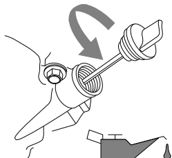
Figure 4-1. Plein d'huile moteur
