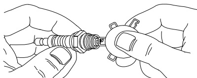
Figure 4-6. Bougie
