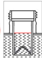
Figura 2-10. Nivel del depósito de combustible interno
