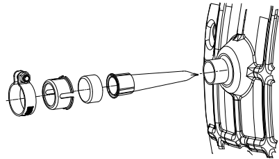
Figure 4-6. Tamis pare-étincelles
